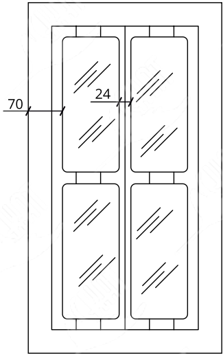
Сечение фасада
